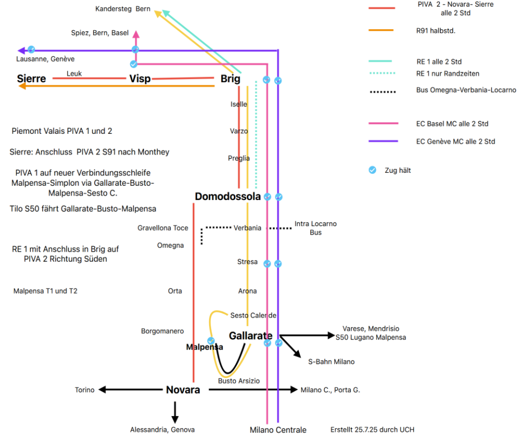
Mögliches Liniennetz nach Abschluss Bauarbeiten Simplon
